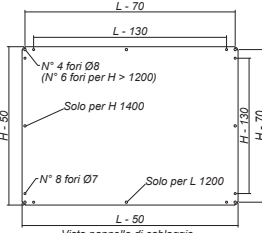
Vista pannello di cablaggio
